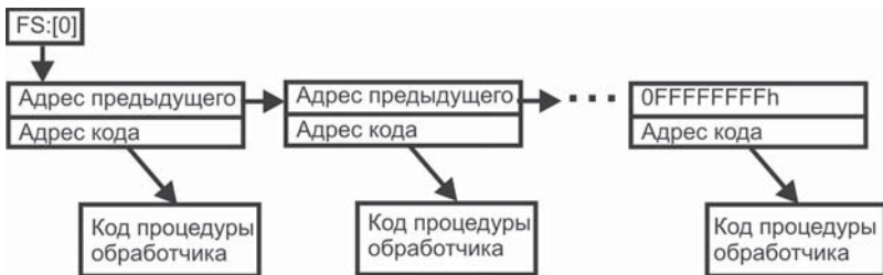
Рис. 4.3 ❖ Цепочка обработчиков исключений
