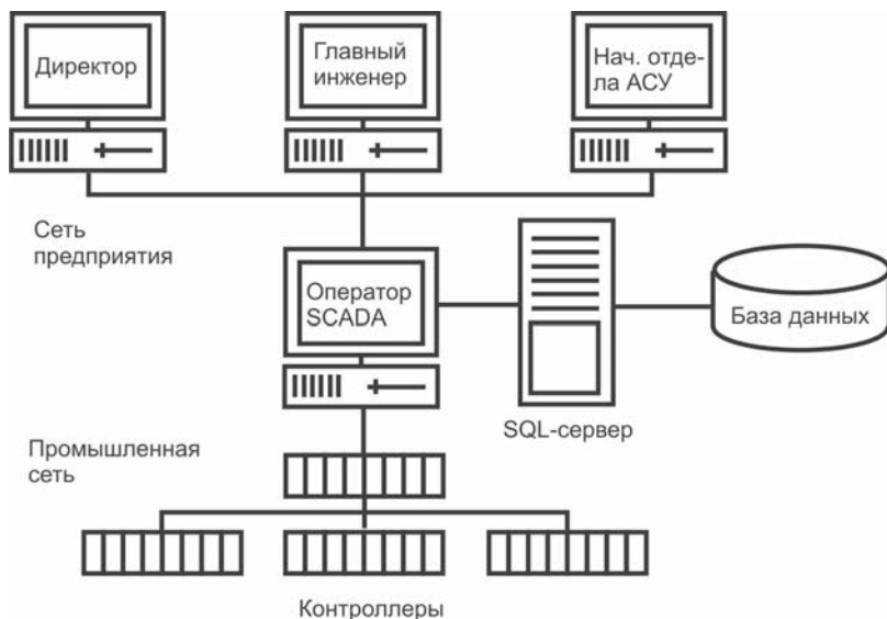
Рис. 7.60 ❖ Типичная структура АСУ ТП
