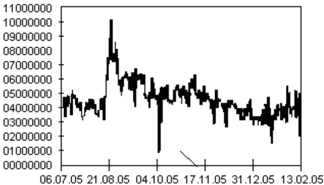
Рис. 7.18 ❖ Сетевой трафик через порт 445 во время эпидемии червя Bozori
