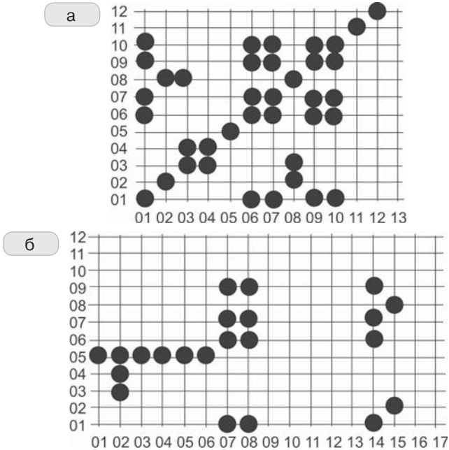
Рис. 7.43 ❖ Сравнение кодов на «близость»: а) близость полиморфного кода с самим собой; б) близость двух копий расшифровщика вируса Vandersnatch
