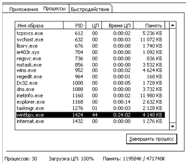
Рис. 6.5 ❖ Процесс червя Vozorg в памяти компьютера
