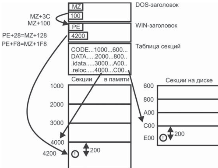
Рис. 4.16 ❖ Схема поиска вируса Varum в файле
