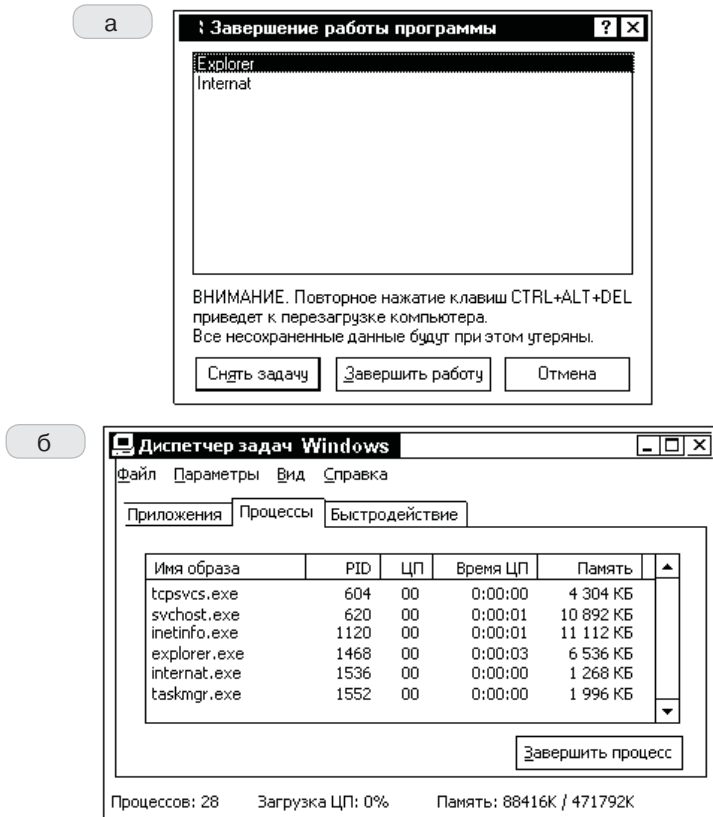
Рис. 4.14 ❖ Менеджеры процессов – TASKMAN и TASKMGR: а) TASKMAN в Windows 9X; б) TASKMGR в Windows NT
