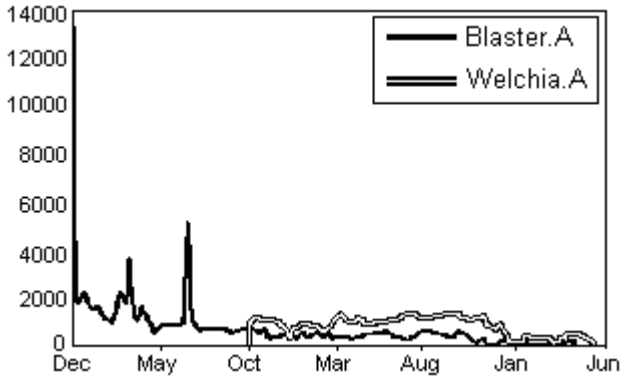
Рис. 7.20 ❖ Подавление червем Welchia эпидемии червя Blaster
