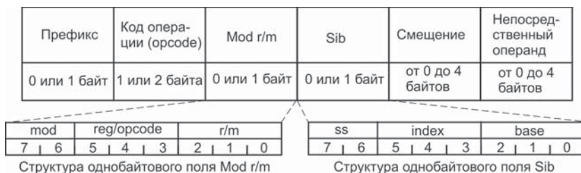
Рис. 7.37 ❖ Структура машинной команды в 32-битовом режиме
