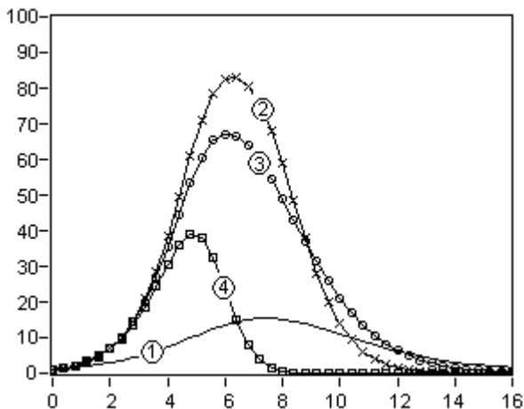
Рис. 7.22 ❖ Кривые размножения сетевых червей, подавляемых «контрчервями»
