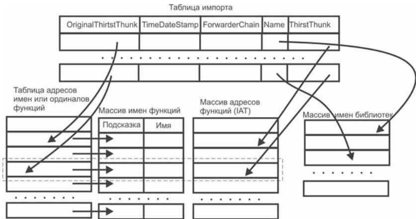
Рис. 4.11 ❖ Организация импорта в PE-программах
