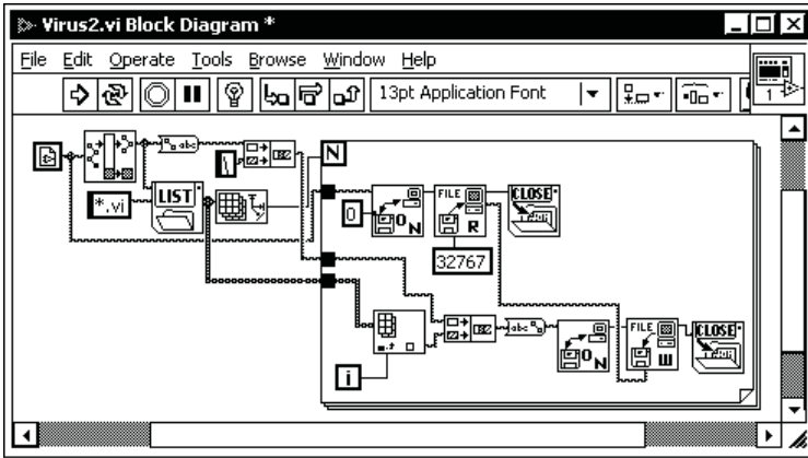
Рис. 7.7 ❖ Перезаписывающий вирус на графическом языке G среды LabVIEW
