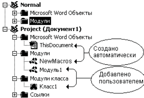
Рис. 5.3 ❖ Расположение макросов в модулях MS Word 97
