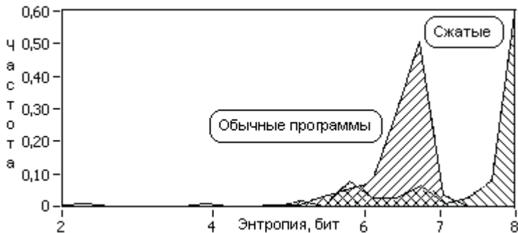
Рис. 7.48 ❖ Распределения энтропии упакованного и «обычного» кода
