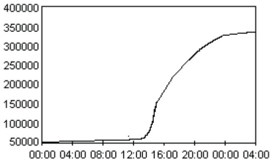
Рис. 7.15 ❖ Динамика размножения червя CodeRed II
