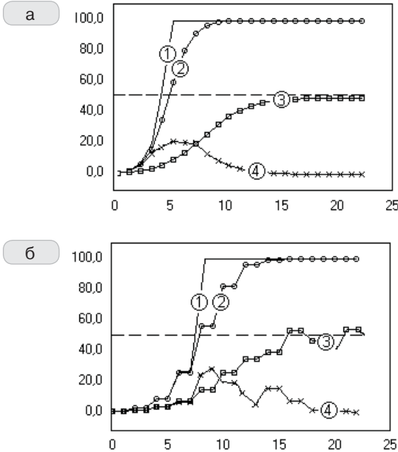
Рис. 7.13 ❖ Кривые размножения мобильных агентов (1 – экспоненциальная SI-модель Мальтуса; 2 – логистическая SI-модель Фергюльста; 3 – SIS-модель; 4 – SIR-модель Кермака-Маккендрика): а) гладкие решения дифференциальных уравнений; б) осциллирующие результаты имитационных экспериментов
