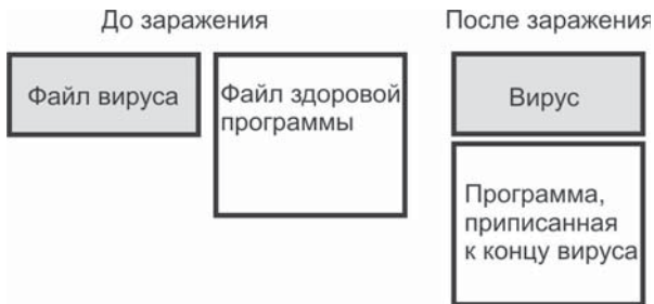
Рис. 3.2 ❖ Принцип заражения, используемый «оверлейными» вирусами
