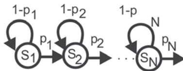
Рис. 7.44 ❖ Марковская цепь
