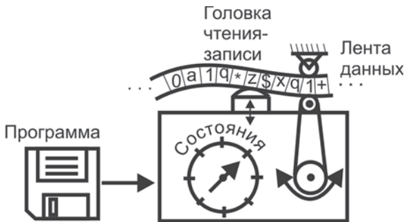
Рис. 7.1 ❖ Машина Тьюринга
