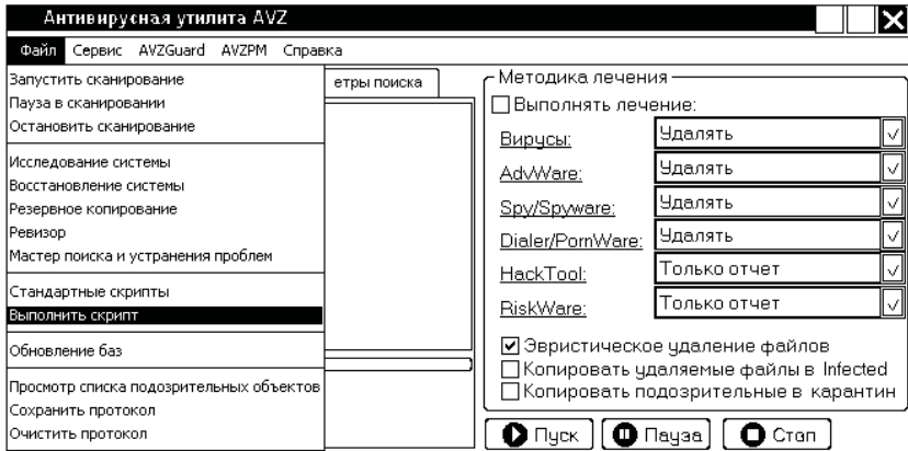
Рис. 6.23 ❖ Антивирус AVZ
