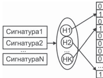
Рис. 7.33 ❖ Фильтр Блума
