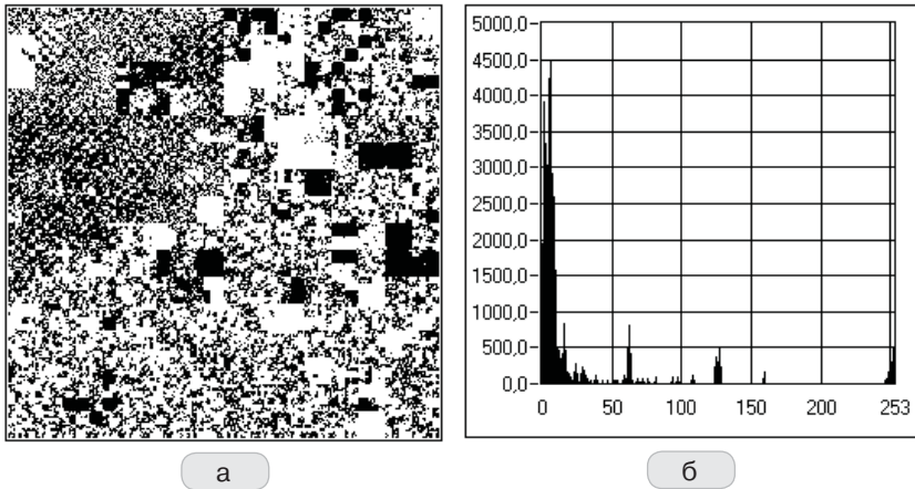
Рис. 7.19 ❖ Неравномерность «живых» IP-адресов в сегментах Интернета: а) типичная «карта» сегмента; б) типичная гистограмма распределения длин непрерывных цепочек
