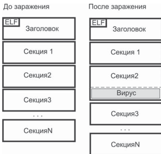
Рис. 7.8 ❖ Схема заражения ELF-программ вирусом Linux.Binom
