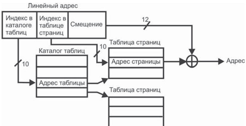
Рис. 4.2 ❖ Страничная адресация
