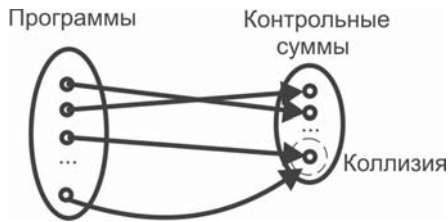
Рис. 7.30 ❖ Сущность «коллизии»
